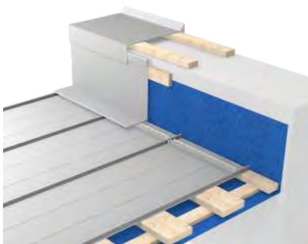
Rys.35 Przykład rozwiązania obróbki przyściennej ogniomuru.
