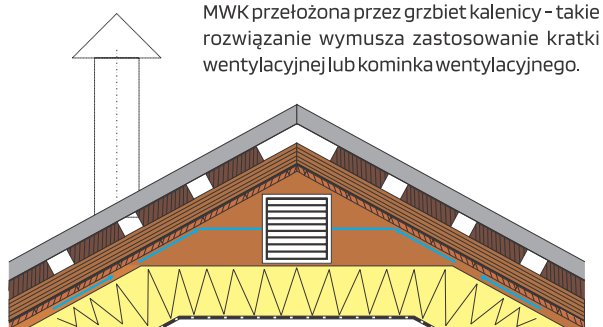
Rys. 6 Przykładowe rozwiązania linii okapu i kalenicy - dach odeskowany + papa.
