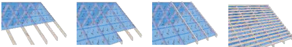
Rys. 7 Kolejne etapy montażu folii, kontrłaty i łąt.
