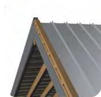
Rys. 29 Montujemy obróbki szczytowe.
