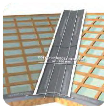
Rys.18 Montaż rynny koszowej.
