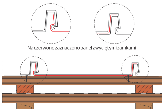
Rys.21 Sposób wycinania zamków.
