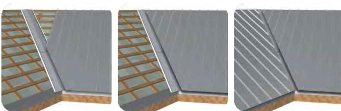
Rys.19 Kolejność montażu paneli przy rynnie koszowej.
