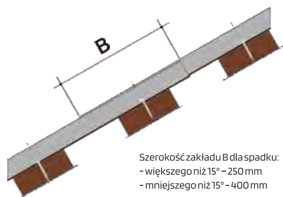
Rys.22 Szerokość zakładu – B.
