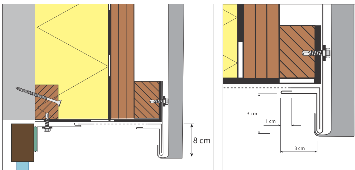
rys.9. Schemat rozwiązania obróbki blacharskiej u dołu lub u góry okna. Rysunek po prawej stronie jest przedstawieniem detalu w zbliżeniu.
