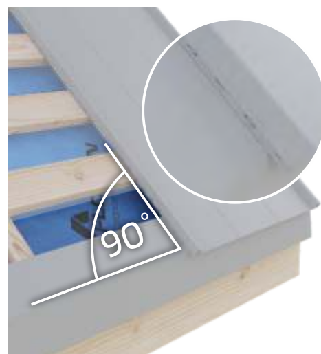
Rys. 12 Panele muszą być układane prostopadłe do okapu. Przy okapie panel mocujemy dwoma wkrętami.
