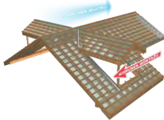
Rys.10 Kierunek montażu przeciwny do kierunku wiatru.
