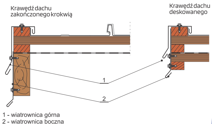
Rys.30 Montaż panela przy desce szczytowej.
