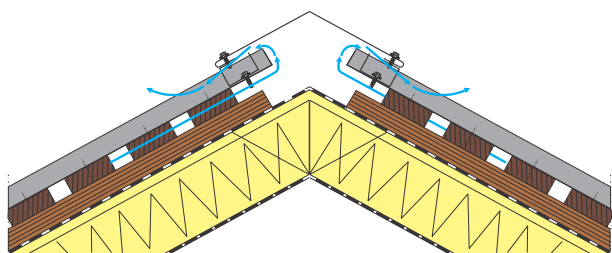
Rys. 5 Przykładowe rozwiązania linii okapu i kalenicy - dach nieodeskowany + folia MWK.
