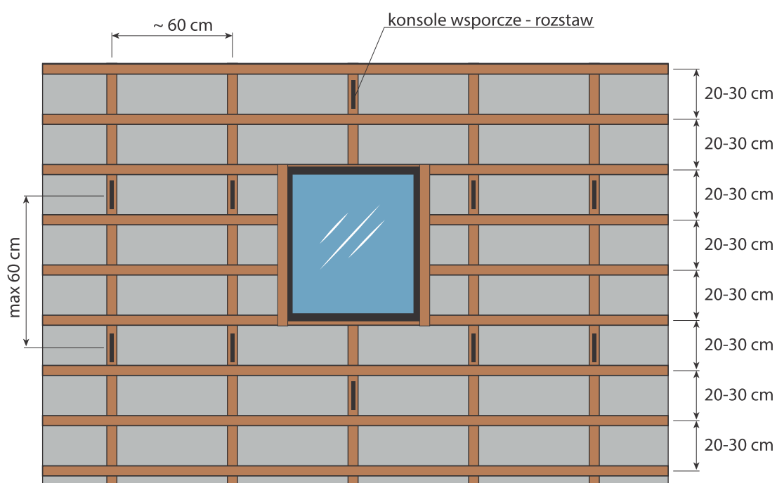
rys 7. Przykładowy rozstaw kontrłat, łat i konsol wsporczych na ścianie.
