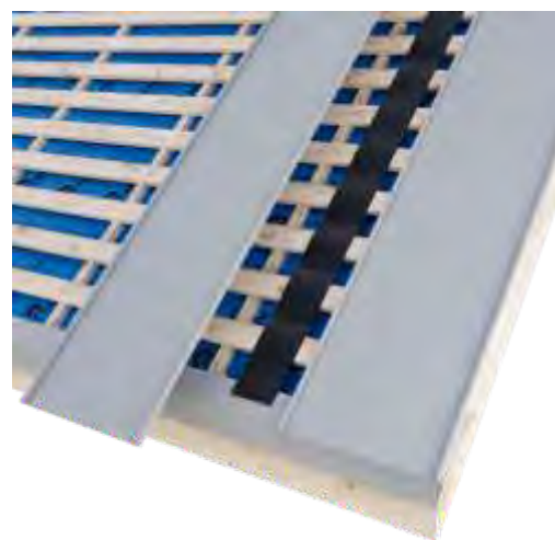
Rys. 13 Taśma wygłuszająca – zalecana pod konstrukcje metalowe.
