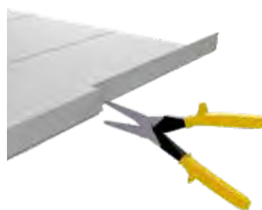
Rys.23 Zamek wycinamy po obydwu stronach panela.
