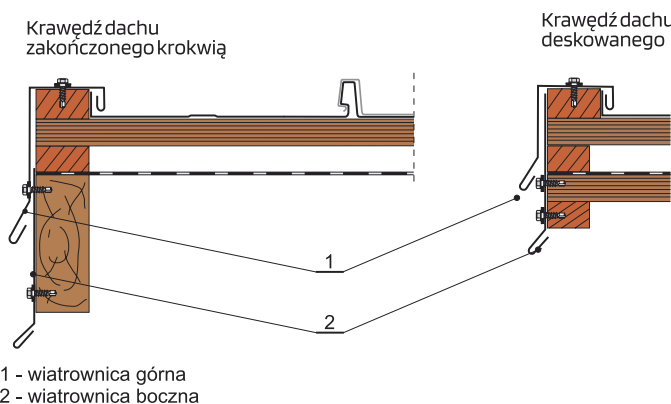
Rys. 29 Montaż panela przy desce szczytowej.
