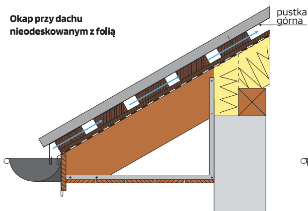
Okap przy dachu wykończonym deskami i papą
