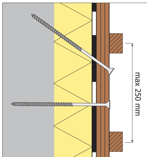
rys. 4. Przekrój podkonstrukcji drewnianej bez wykorzystania konsol wsporczych
