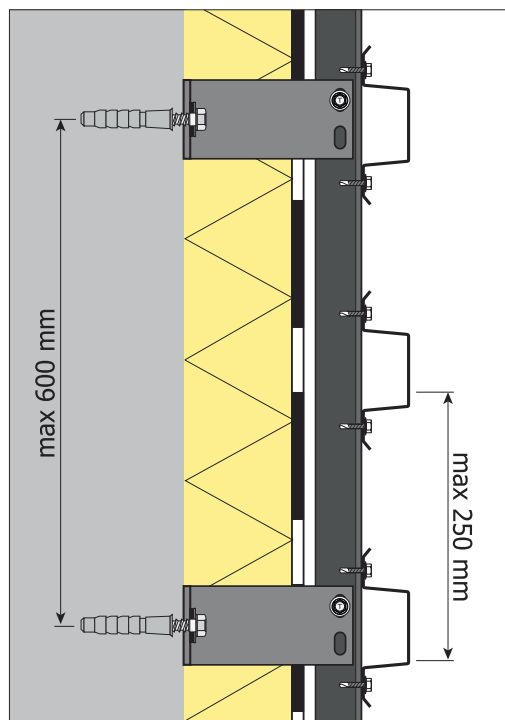
rys. 3. Przekrój podkonstrukcji stalowej z wykorzystaniem konsol wsporczych.
