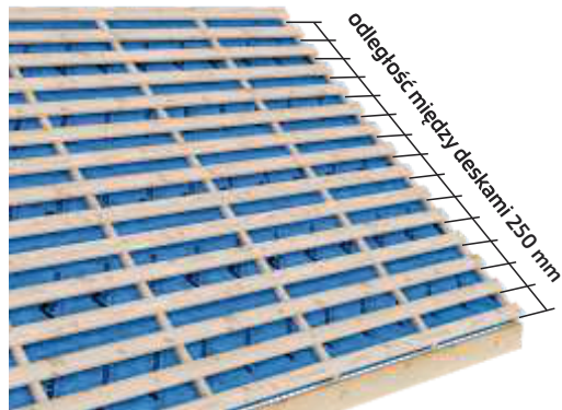
Rys. 2 Rozmieszczenie desek na dachu. Rozstaw powinien wynosić co 250 mm - mierzone od tych samych krawędzi.
