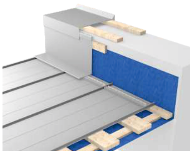
Rys.34 Przykład rozwiązania obróbki przyściennej ogniomuru.
