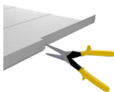
Rys.22 Zamek wycinamy po obydwu stronach panela.
