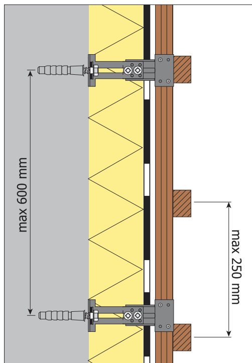
rys. 2. Przekrój podkonstrukcji drewnianej z wykorzystaniem konsol wsporczych.
