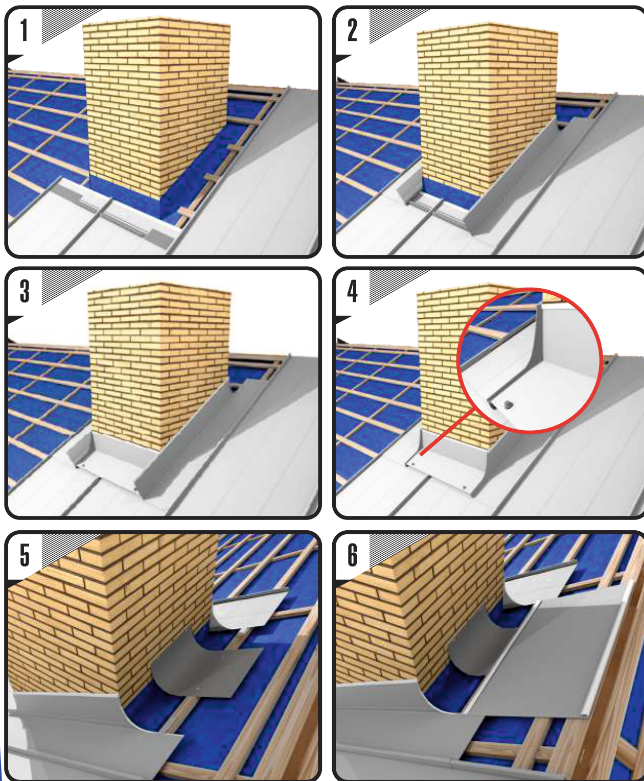
Rys.36 Etapy montażu obróbki komina
