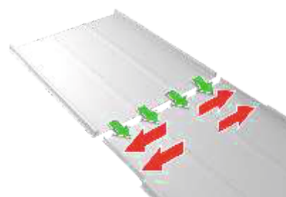
Rys.23 Dopasowujemy panele do siebie – zamek należy rozbić o 1 mm na zewnątrz.
