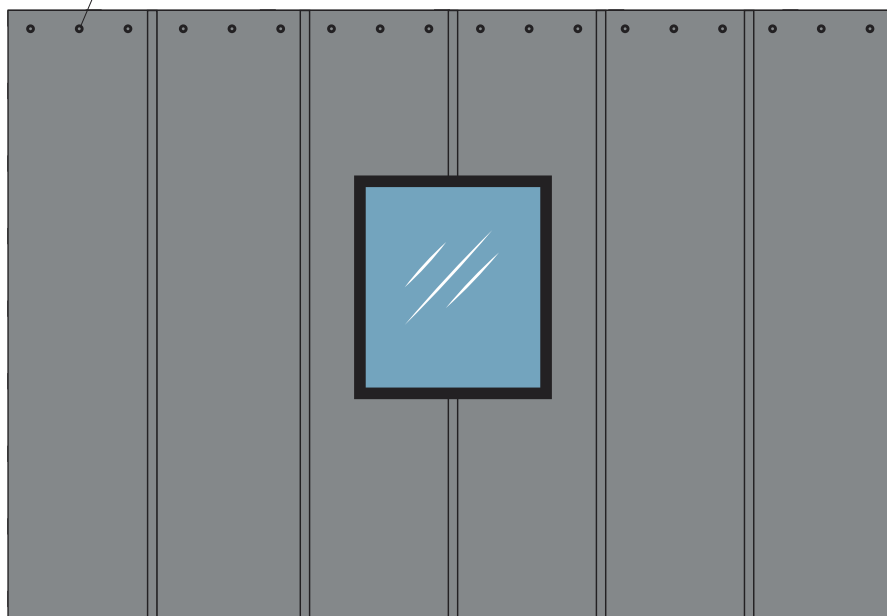
rys 6. Przykładowe rozmieszczenie łączników na ścianie. Łączniki powinny być mocowane do listwy podgąsiorowej.
