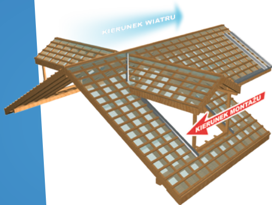
Rys. 10 Kierunek montażu przeciwny do kierunku wiatru
