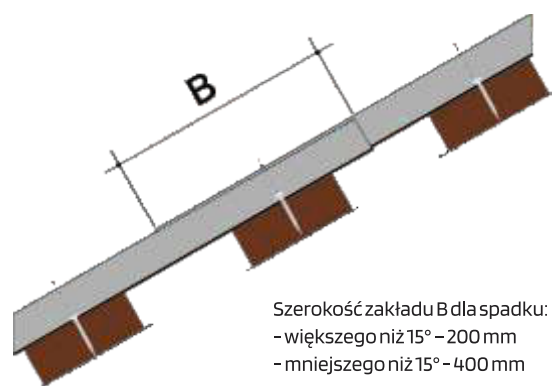
Rys.21 Szerokość zakładu - B.
