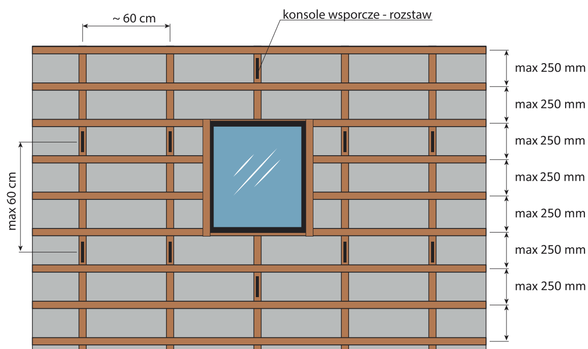
rys6. Przykładowy rozstaw kontrłat, łat i konsol wsporczych na ścianie.
