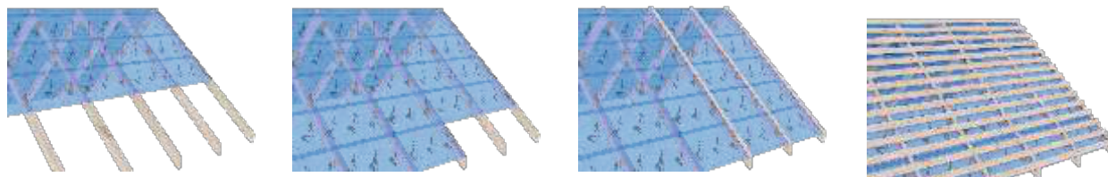
Rys. 7 Kolejne etapy montażu folii, kontrłaty i łat.
