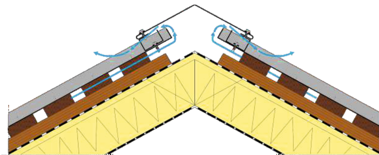
Rys.32 Zastosowanie kalenicy prostej przy kryciu wstępnym membraną.
