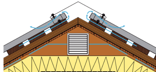
Rys. 6 Przykładowe rozwiązania linii okapu i kalenicy - dach odeskowany+papa.
