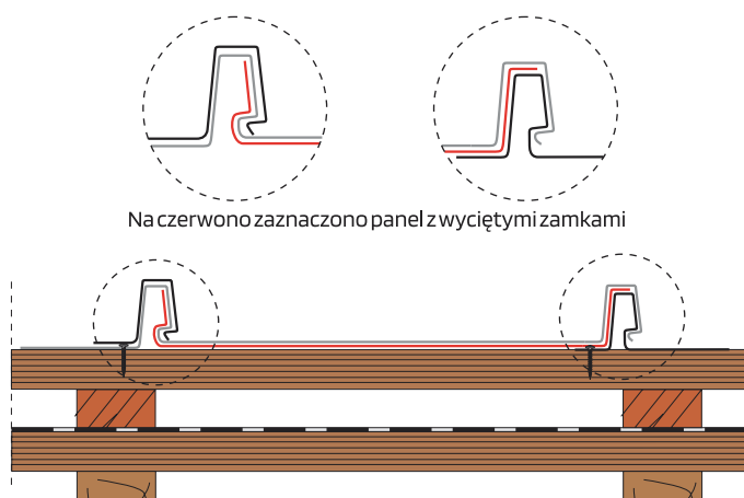
Rys.20 Sposób wycinania zamków.
