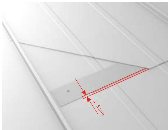
Rys. 16 Połączenie paneli na obcą listwę.
