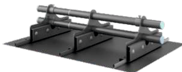
Rys.35 Przykład zastosowania bariery śniegowej.
