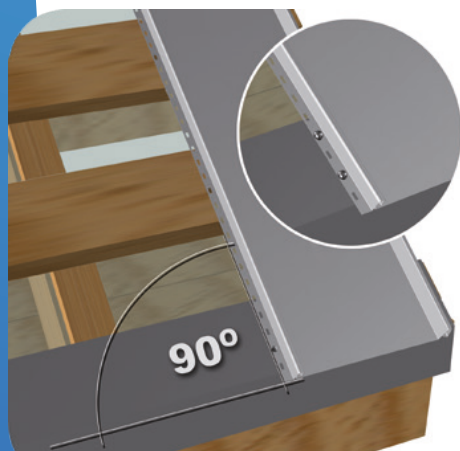
Rys. 11 Panele muszą być układane prostopadłe do okapu. Przy okapie panel mocujemy dwoma wkrętami
