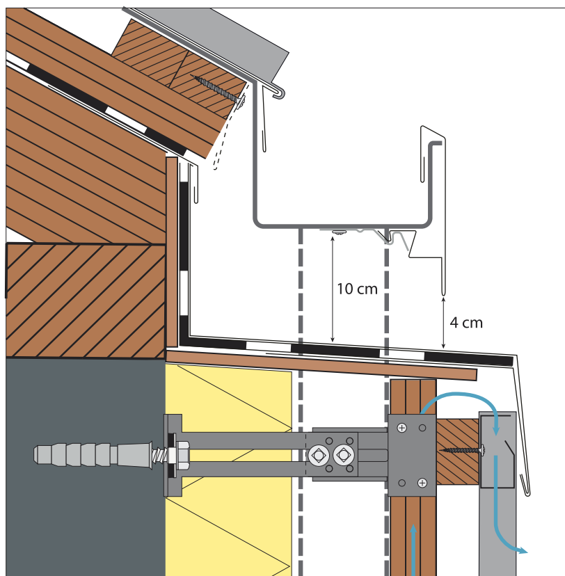
rys.13. Schemat obróbek blacharskich przy rynnie w systemie ukrytym.
