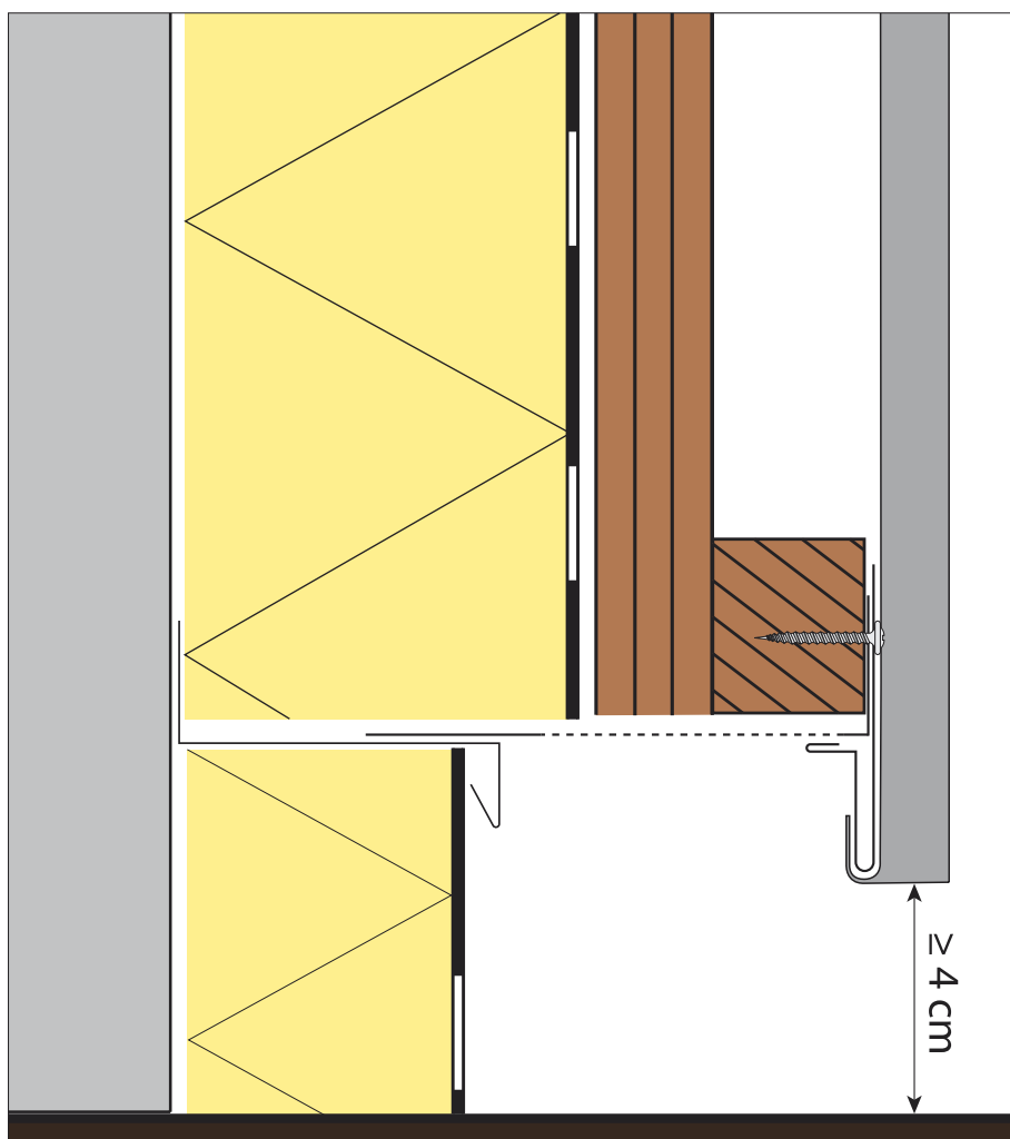
rys 7. Schemat rozwiązania obróbki blacharskiej u dołu ściany (od podłoża).
