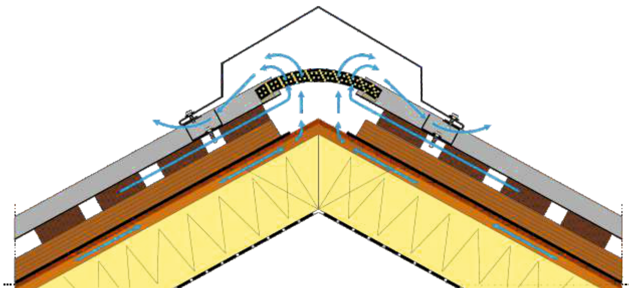
Rys.33 Zastosowanie kalenicy stożkowej przy kryciu wstępnym z papą wraz z przykładem zabezpieczenia „pustki dolnej” przed zawiewaniem deszczu i śniegu
