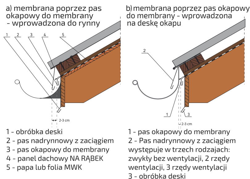
Rys. 8 Sposoby mocowania FWK na okapie oraz instalacja pasa nadrynnowego i nadrynnowego.
