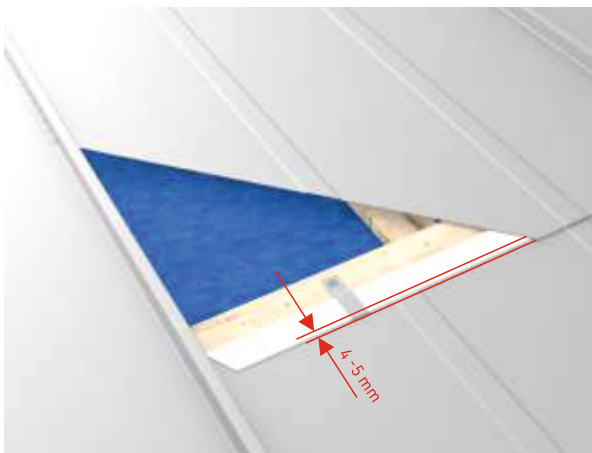
Rys. 15 Połączenie paneli na zacięciu.
