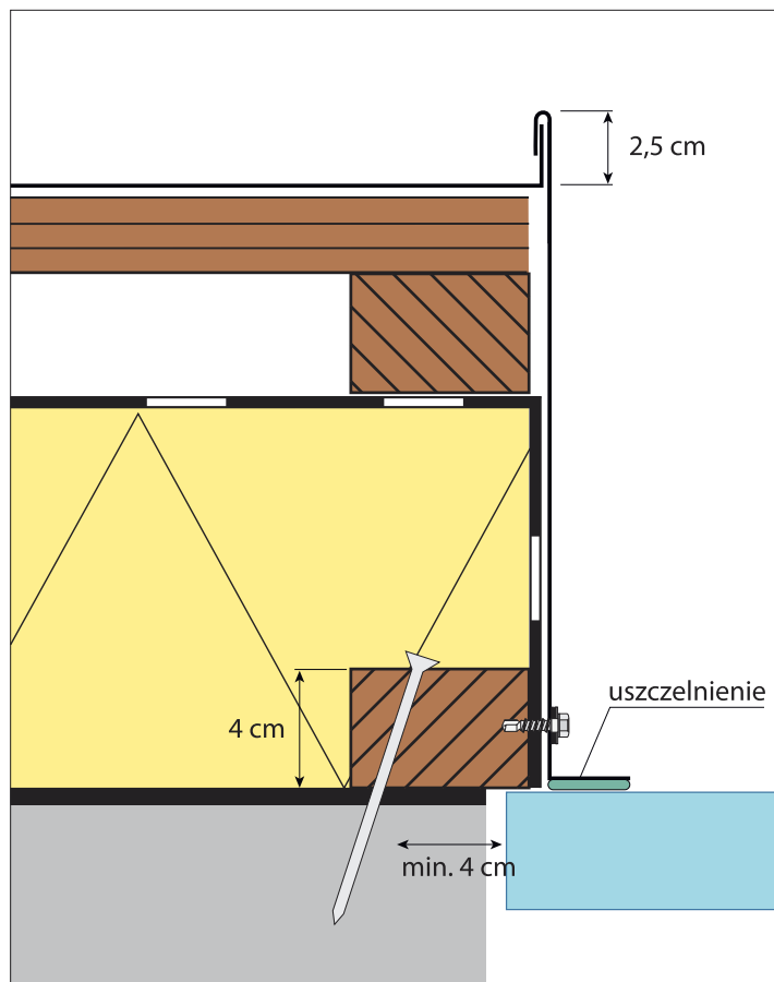
rys. 8. Schemat rozwiązania obróbki blacharskiej przy boku okna.
