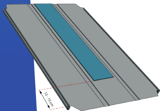
Rys. 13 Taśma wygłuszająca - zalecana na każdy rodzaj podkonstrukcji, w szczególności metalowe.
