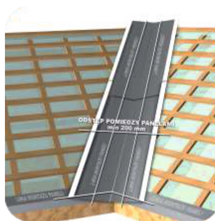
Rys. 17 Montaż rynny koszowej.
