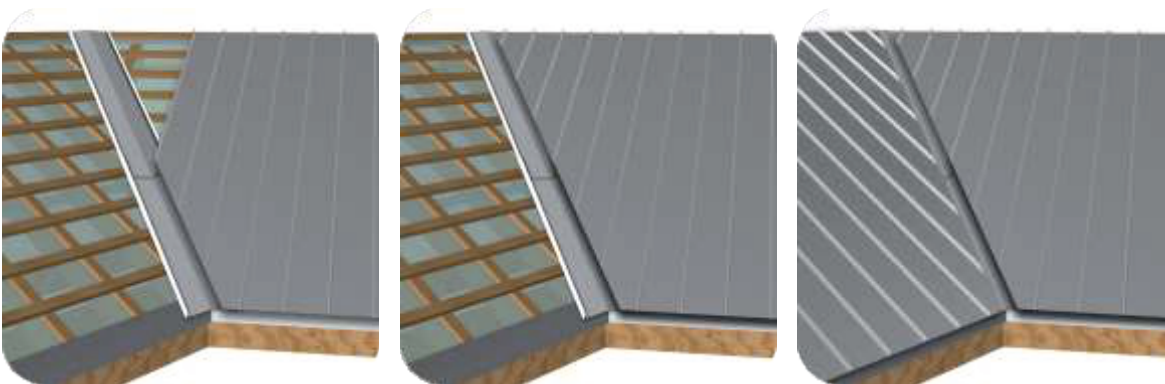
Rys. 18 Kolejność montażu paneli przy rynnie koszowej.
