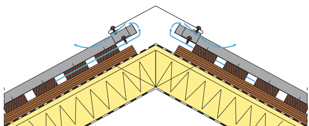
Rys. 5 Przykładowe rozwiązania linii okapu i kalenicy - dach niedeskowany+folia MWK.
